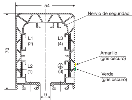
A - A KBH-4 polos
